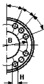
Bride de palier / Mâchoire à bride
