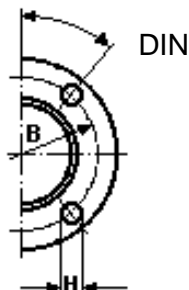
Bride de palier / Mâchoire à bride
