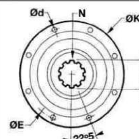
FIG 5 : DIN 8 TROUS
