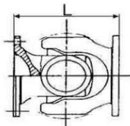
FIG 2 : DIN 6 TROUS
