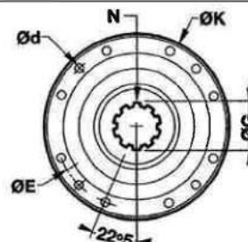
FIG 3 : SAE 12 TROUS
