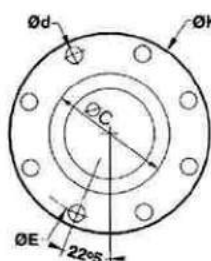
FIG 3 : DIN 8 TROUS
