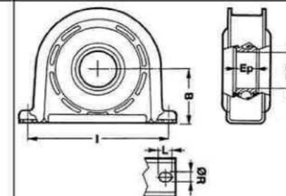
Schéma + dimensions
