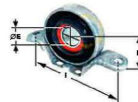
Schéma + dimensions
