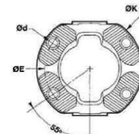
FIG 5 : DENT. 4 TROUS
