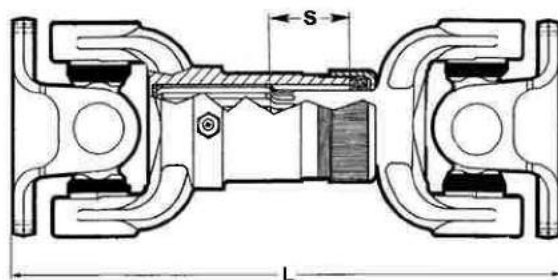
FIG 1 : DIN 4 TROUS
