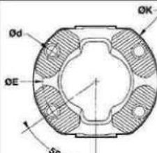
FIG 5 : DENT. 4 TROUS
