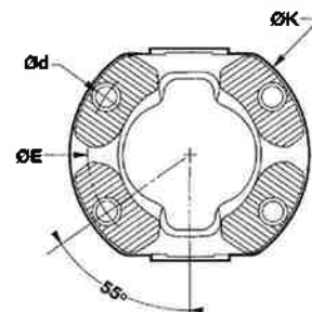
FIG 10 : DENTURE 4 TROUS
