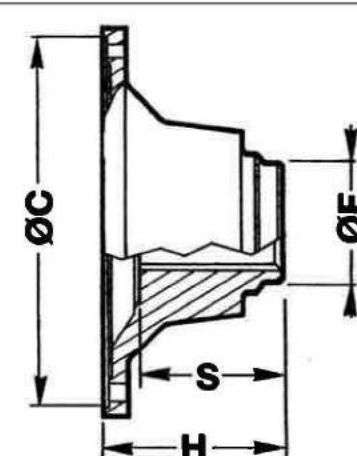
FIG B : bride palier DIN
