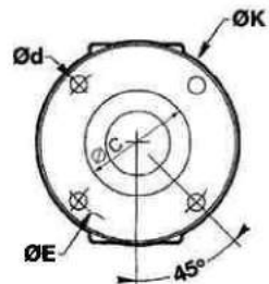
FIG 1 : DIN 4 TROUS
