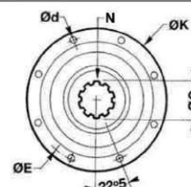
FIG 5 : DIN 8 TROUS
