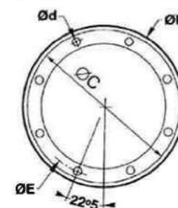
FIG 6 : SAE 12 TROUS
