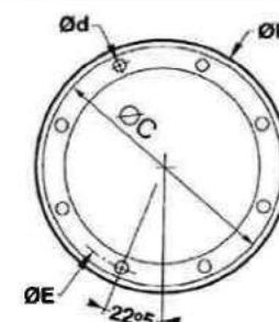
FIG 6 : SAE 12 TROUS
