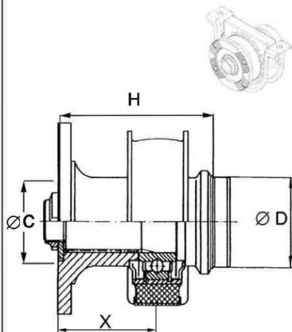
FIG 2 : SAE 8 TROUS
