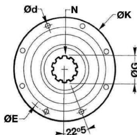
FIG 5 : DIN 8 TROUS
