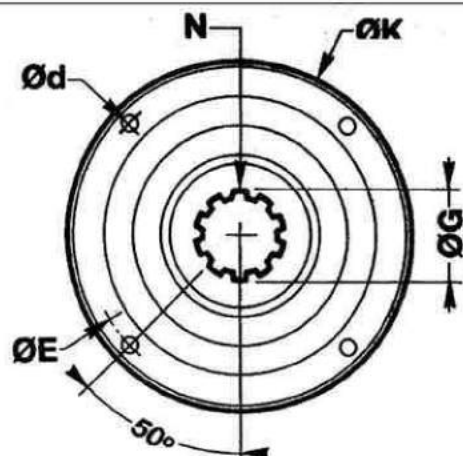
FIG 4 : DENT 4 TROUS
