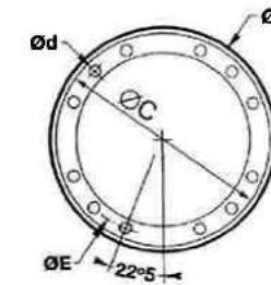
FIG 6 : SAE 12 TROUS
