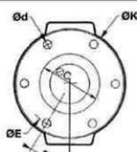
FIG 2 : DIN 6 TROUS
