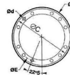
FIG 6 : SAE 12 TROUS
