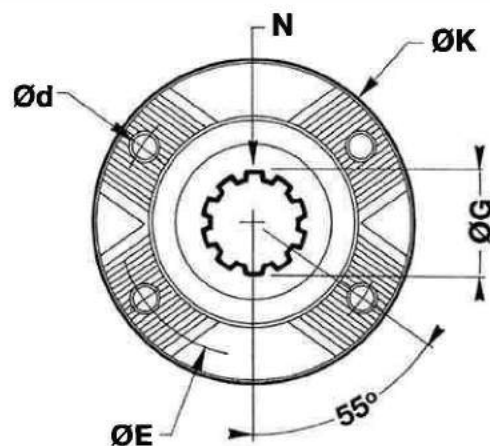
FIG 4 : DENT 4 TROUS
