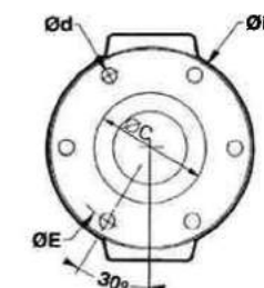
FIG 3 : DIN 8 TROUS
