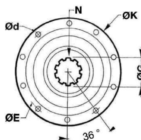
FIG 6 : DIN 10 TROUS
