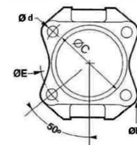
FIG 7 : SAE 8 TROUS
