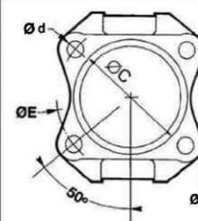
FIG 7 : SAE 8 TROUS
