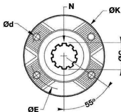
FIG 4 : DENT 4 TROUS
