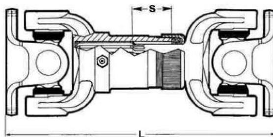
FIG 1 : DIN 4 TROUS
