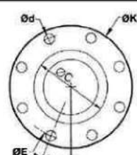
FIG 3 : DIN 8 TROUS
