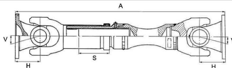
FIG 2 : SAE 12 TROUS
