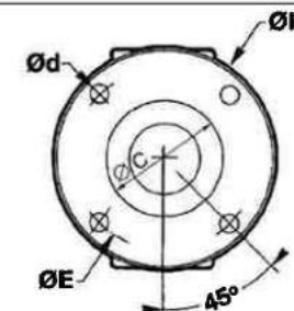
FIG 2 : DIN 6 TROUS
