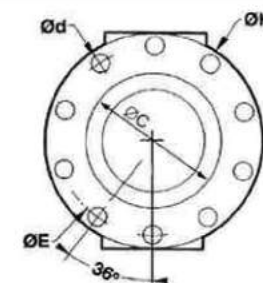
FIG 5 : DIN 10
