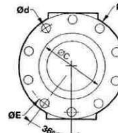
FIG 4 : DIN 10 TROUS
