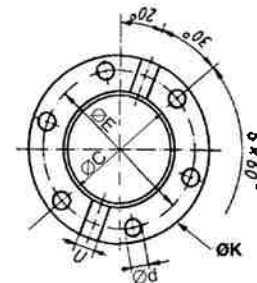
FIG 12 : UNIMOG 6 TROUS
