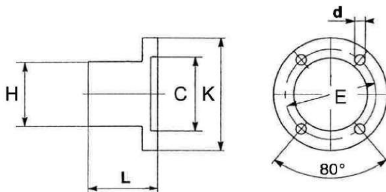
FIG C : CONTRE BRIDE DIN
