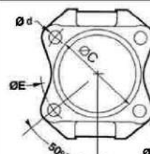
FIG 6 : SAE 4 TROUS
