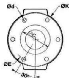
FIG 2 : DIN 6 TROUS
