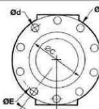
FIG 4 : DIN 10 TROUS
