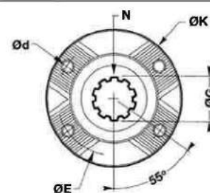
FIG 4 : DENT. 4 TROUS
