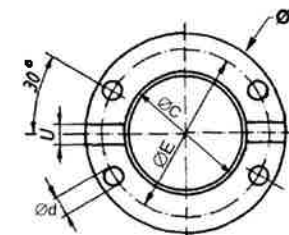
FIG 11 : UNIMOG 4 TROUS
