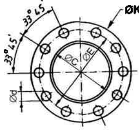
FIG 9 : DIN 10 TROUS DESAXE
