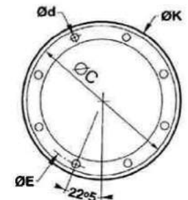
FIG 6 : SAE 12 TROUS
