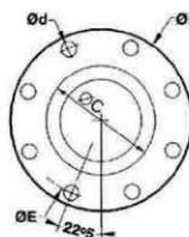
FIG 3 : DIN 8 TROUS
