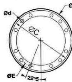
FIG 3 : SAE 12 TROUS
