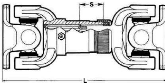
FIG 1 : DIN 4 TROUS
