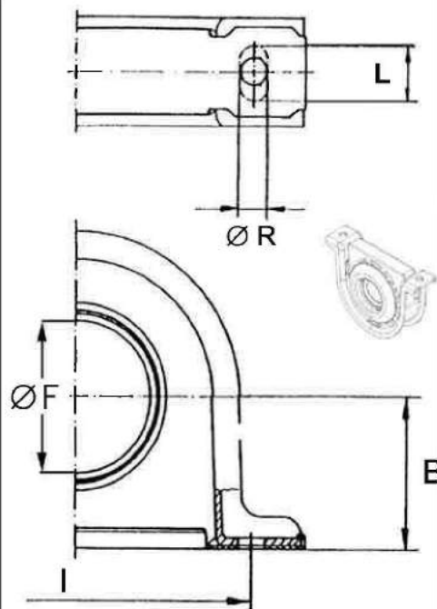
FIG 1 : SAE 4 TROUS
