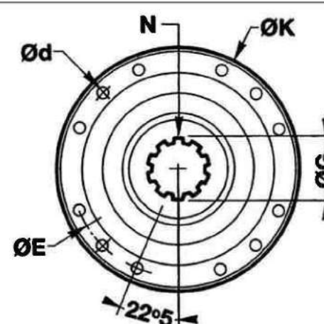
FIG 6 : DIN 10 TROUS
