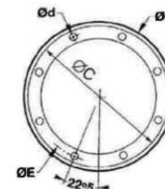
FIG 6 : SAE 12 TROUS
