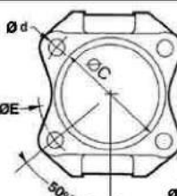
FIG 6 : SAE 4 TROUS
