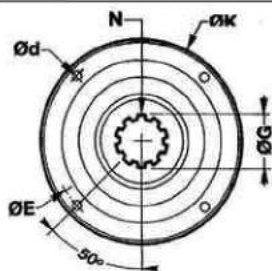
FIG 1 : SAE 4 TROUS
