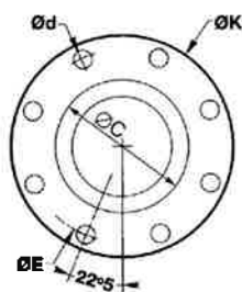
FIG 7 : DIN 8 TROUS
