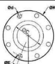
FIG 3 : DIN 8 TROUS
