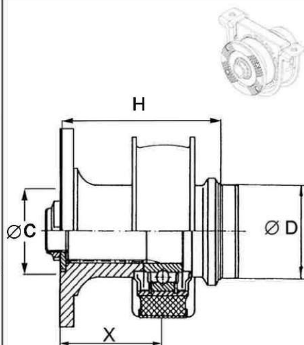
FIG 2 : SAE 8 TROUS
