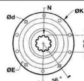
FIG 6 : DIN 10 TROUS
