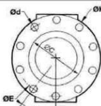
FIG 4 : DIN 10 TROUS
