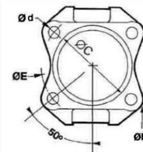
FIG 8 : SAE 4 TROUS
