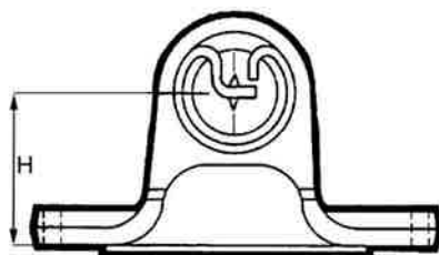
FIG 1 : SAE 4 TROUS
