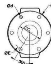
FIG 5 : DIN 6 TROUS
