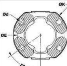
FIG 5 : DENT. 4 TROUS
