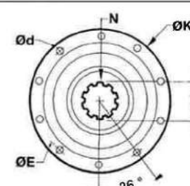
FIG 6 : DIN 10 TROUS
