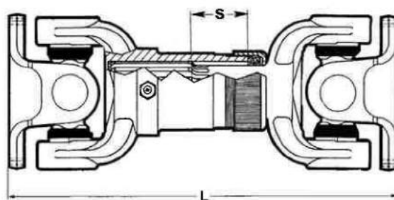
FIG 1 : DIN 4 TROUS
