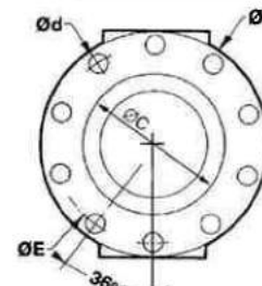
FIG 4 : DIN 10 TROUS
