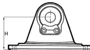
FIG 4 : SAE 12 TROUS
