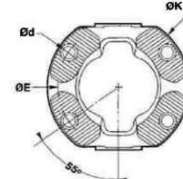
FIG 5 : DENT. 4 TROUS
