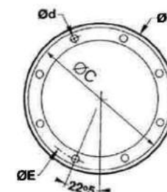
FIG 7 : SAE 8 TOUS
