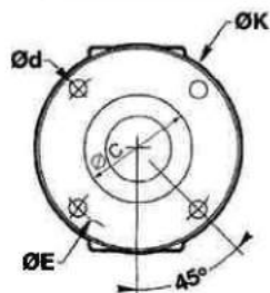
FIG 1 : DIN 4 TROUS
