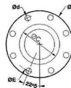
FIG 3 : DIN 8 TROUS
