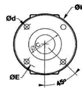
FIG 11 : UNIMOG 4 TROUS
