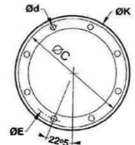
FIG 6 : SAE 12 TROUS
