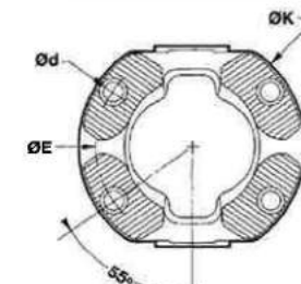
FIG 5 : DENT. 4 TROUS
