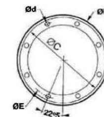
FIG 6 : SAE 12 TROUS
