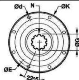
FIG 2 : SAE 8 TROUS
