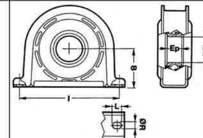
Schéma + dimensions
