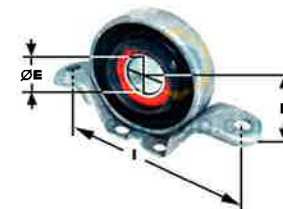
Schéma + dimensions
